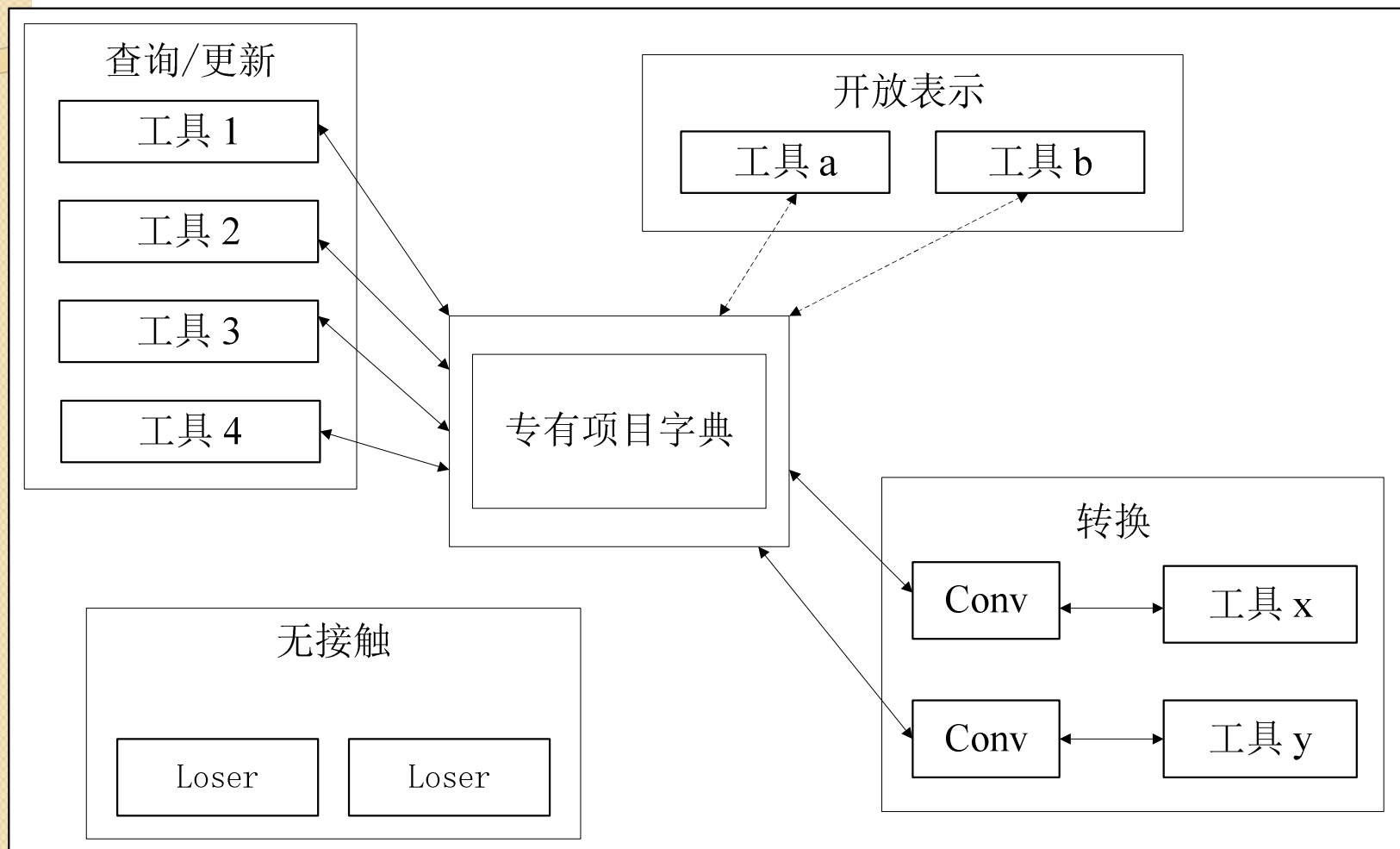
图4-23基于仓库风格的Eclipse软件开发环境
